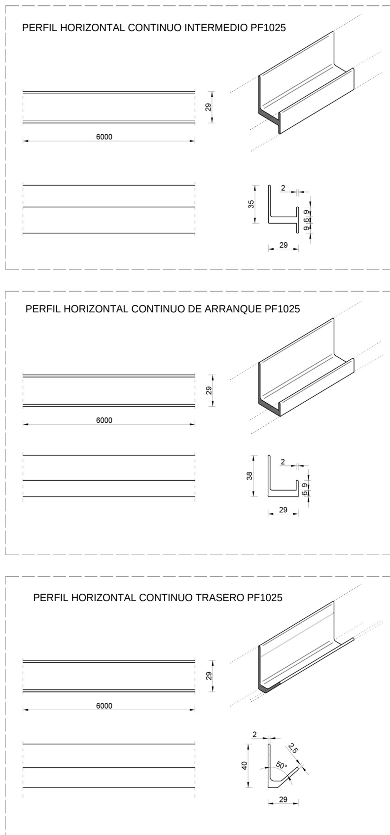
FIGURA 6-B. PERFIL HORIZONTAL OCULTO Y CONTINUO - PF1025 CONTINUO
