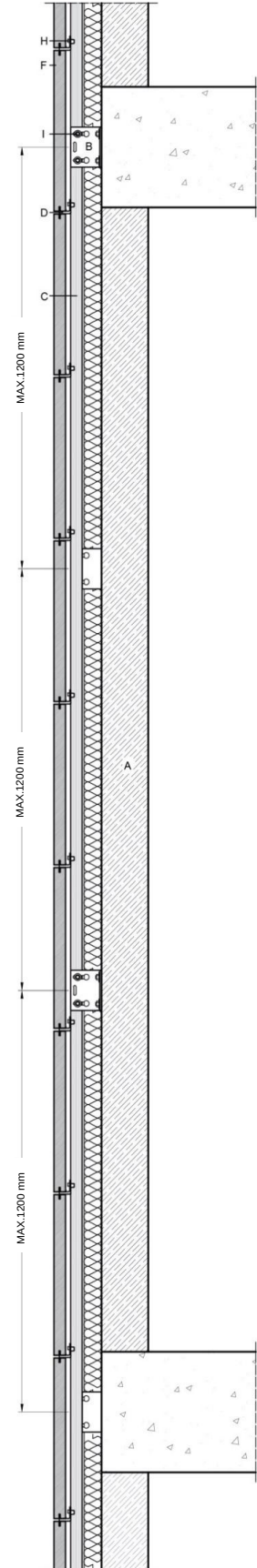
FIGURA 8. SECCIÓN VERTICAL
