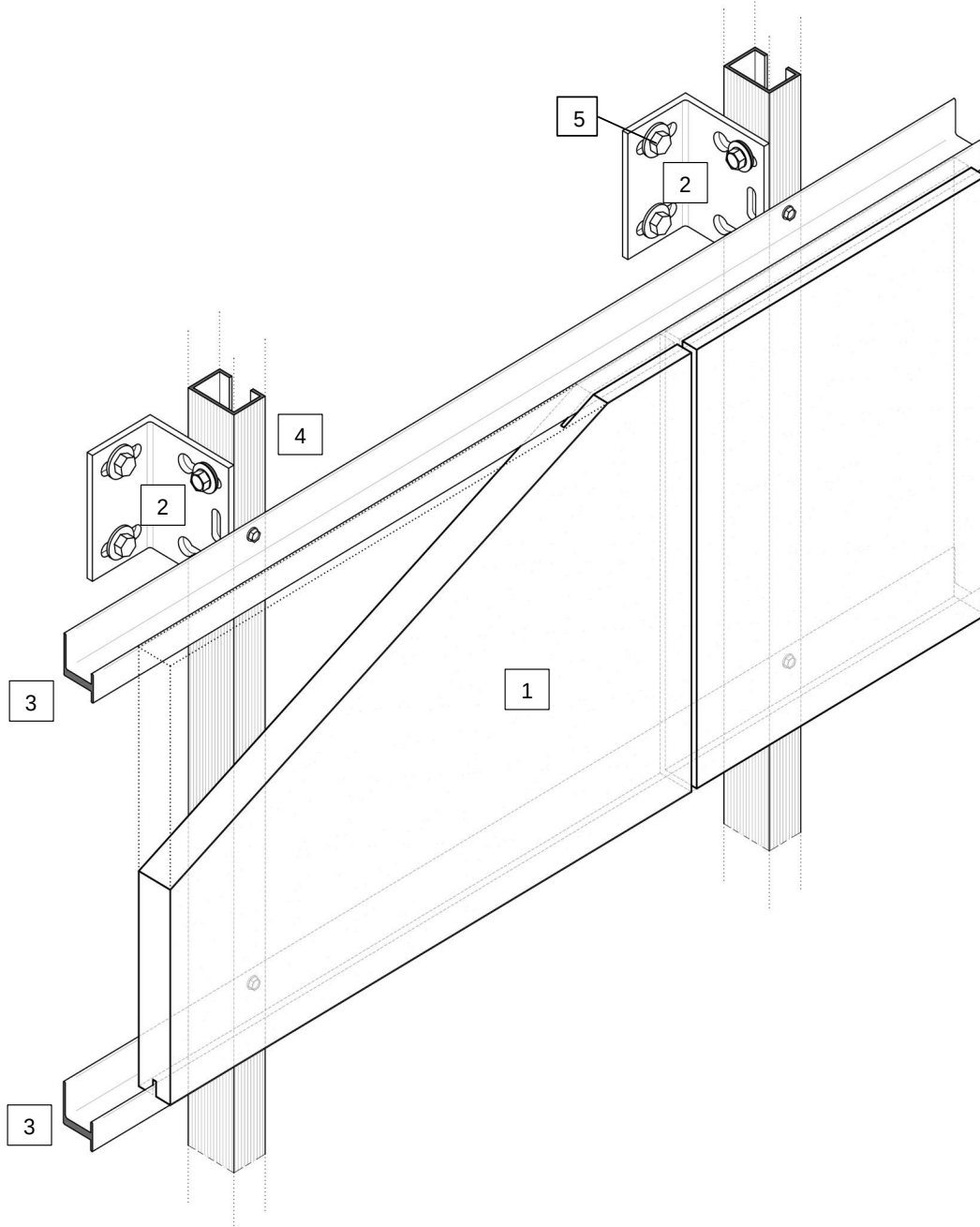
FIGURA 1-B. PF 1025 CONTINUO – PERFIL HORIZONTAL OCULTO Y CONTINUO
