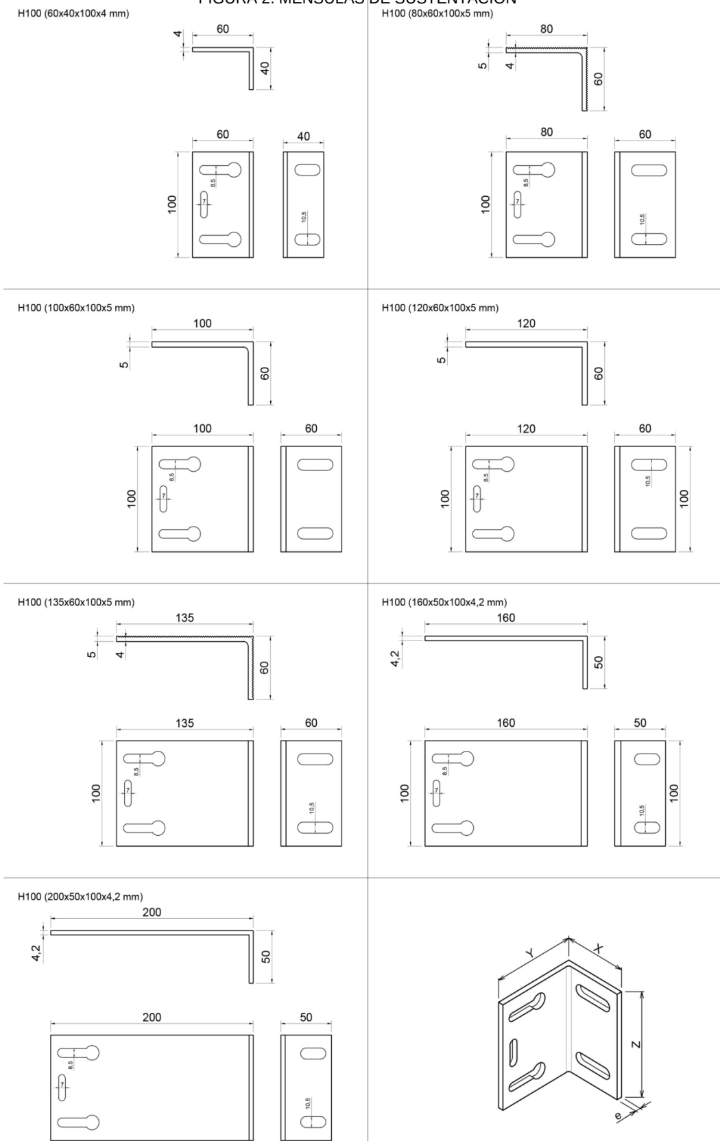
FIGURA 2. MÉNSULAS DE SUSTENTACIÓN
