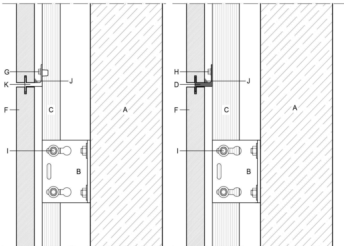
FIGURA 12. DETALLE DEL SISTEMA DE SUBESTRUCTURA Y FIJACIONES – SECCIÓN HORIZONTAL FIGURA 12-A. PF 1025 DISCONTINUO FIGURA 12-B. PF 1025 CONTINUO
