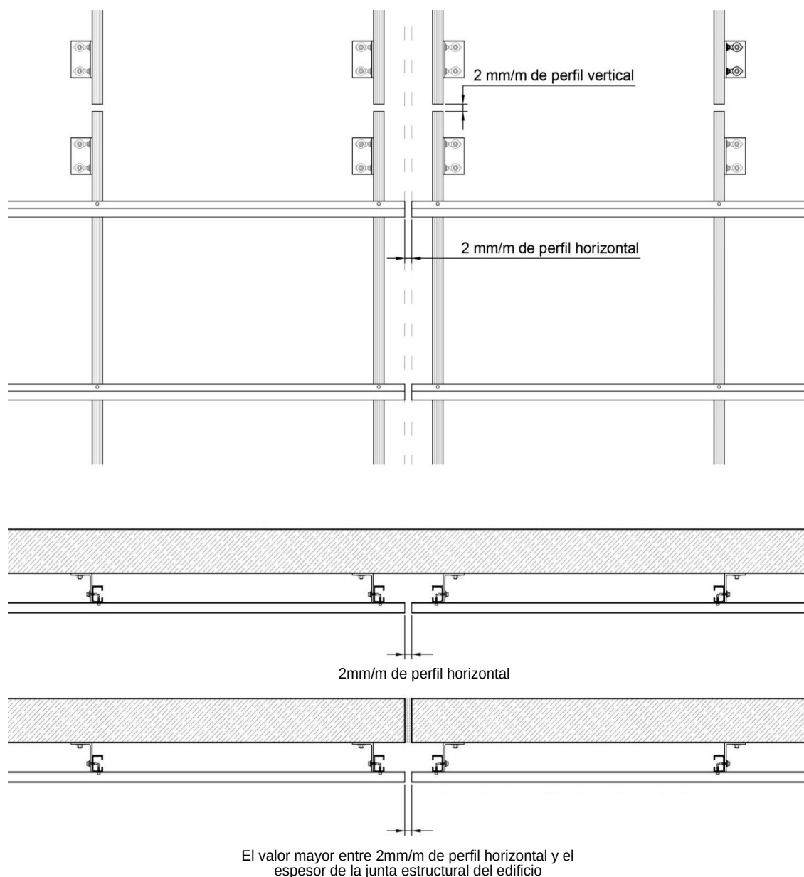
FIGURA 9. DETALLE DE LAS JUNTAS ENTRE PERFILES HORIZONTAL Y PERFILES VERTICALES
