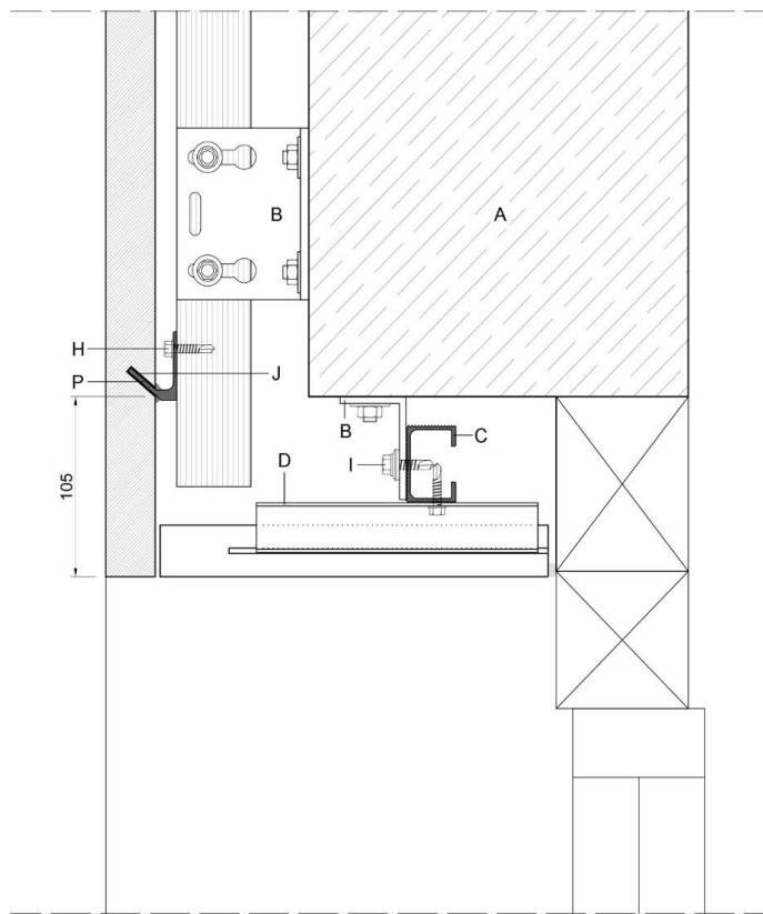
FIGURA 17. DETALLE DE VENTANA CON PERFIL HORIZONTAL TRASERO PF1025 – SECCIÓN VERTICAL
