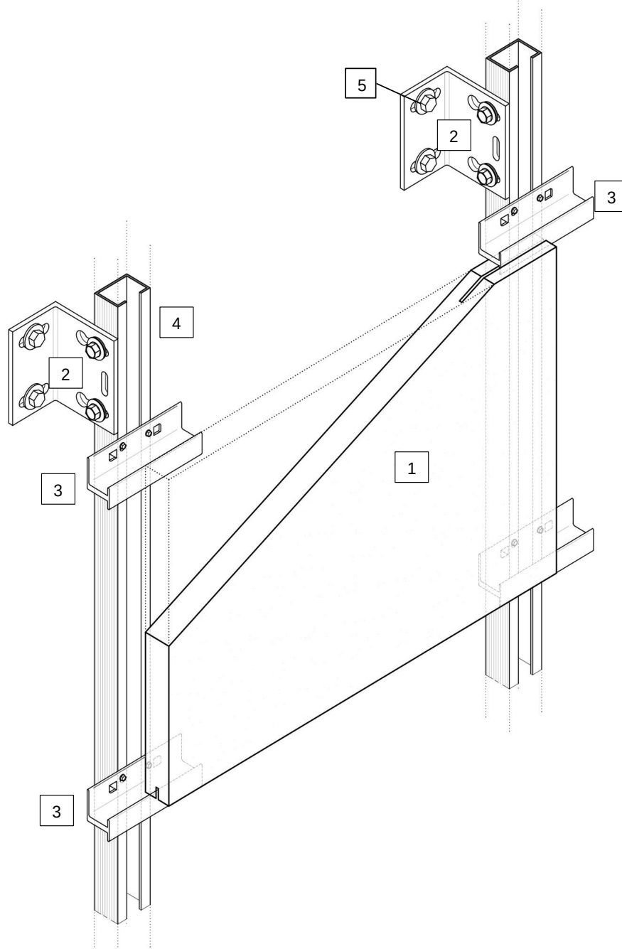
FIGURA 1-A. PF 1025 DISCONTINUO – FIJACIÓN OCULTA Y PUNTUAL
