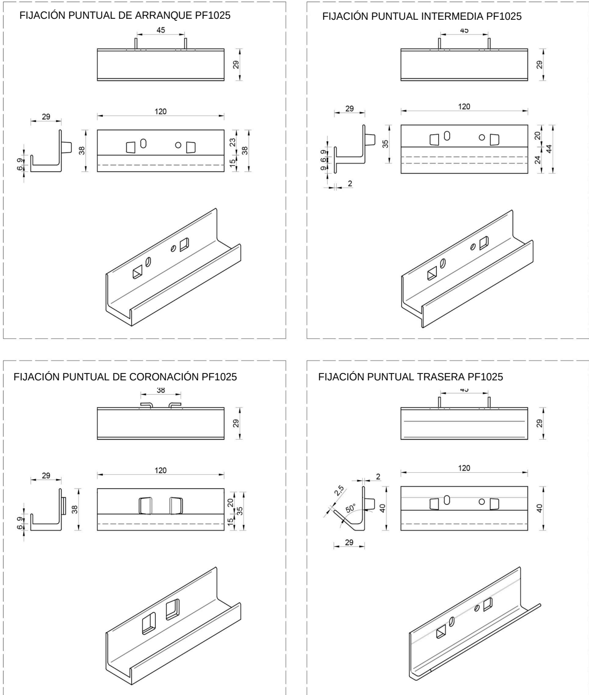
FIGURA 6-A. FIJACIÓN PUNTUAL Y OCULTA - PF1025 DISCONTINUO
