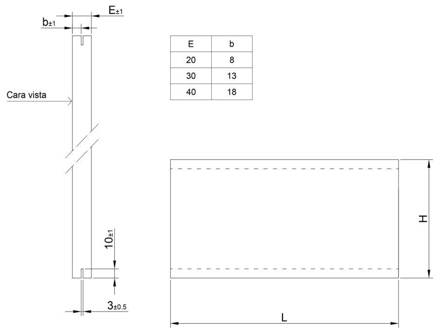
FIGURA 10-A. ELEMENTO DE REVESTIMIENTO GENÉRICO CON RANURADO ESTANDAR
