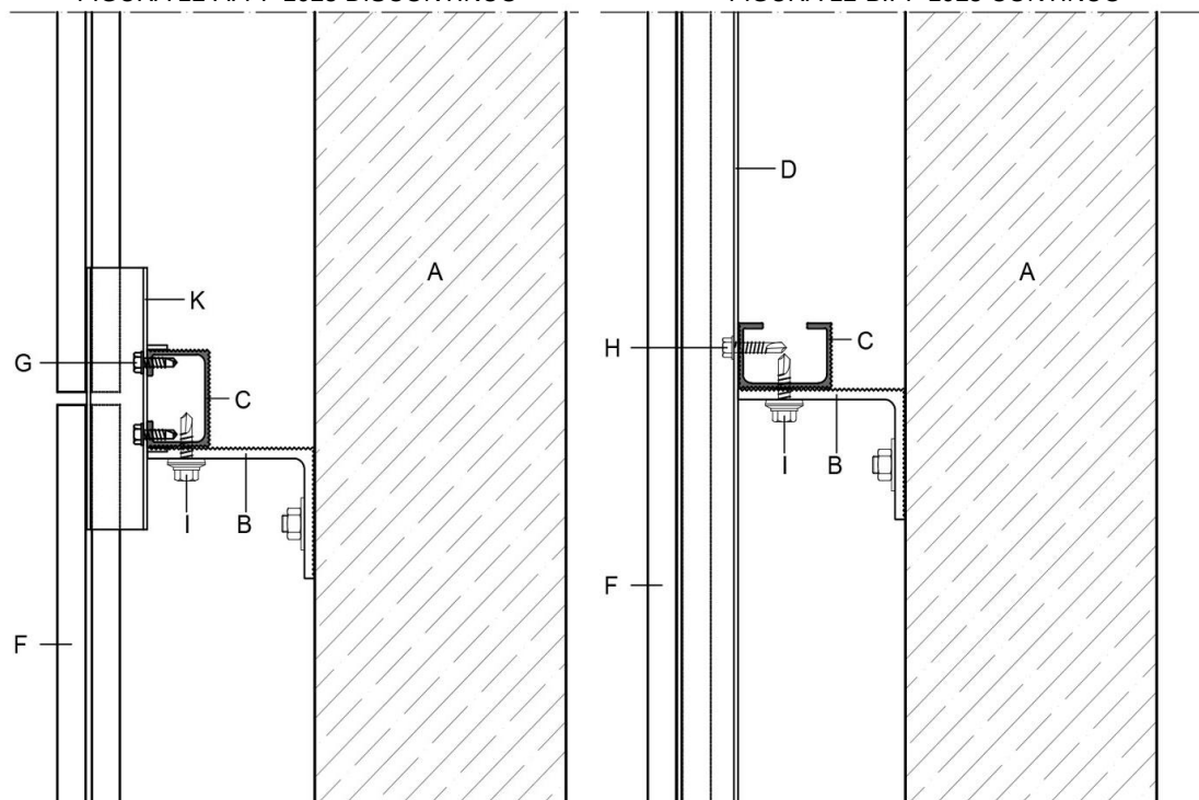
FIGURA 12. DETALLE DEL SISTEMA DE SUBESTRUCTURA Y FIJACIONES – SECCIÓN HORIZONTAL FIGURA 12-A. PF 1025 DISCONTINUO FIGURA 12-B. PF 1025 CONTINUO
