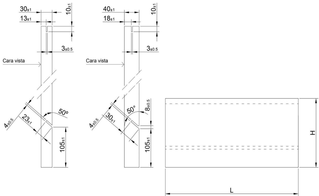
FIGURA 10-B. ELEMENTO DE REVESTIMIENTO GENÉRICO CON RANURADO TRASERO (No disponible para elementos de revestimiento con espesor E<30mm)
